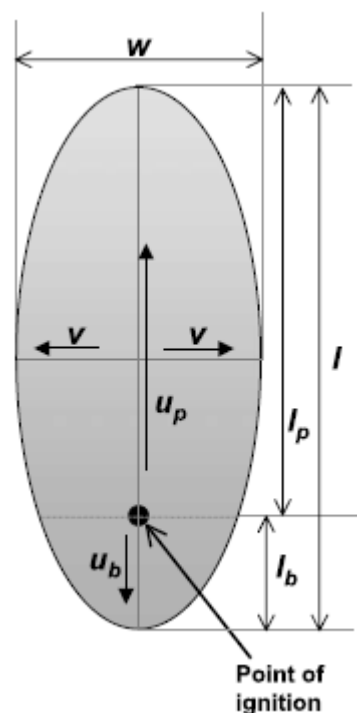
Figura 8 - Espalhamento do Fogo de acordo com o Modelo Arora e Boer (2005)
